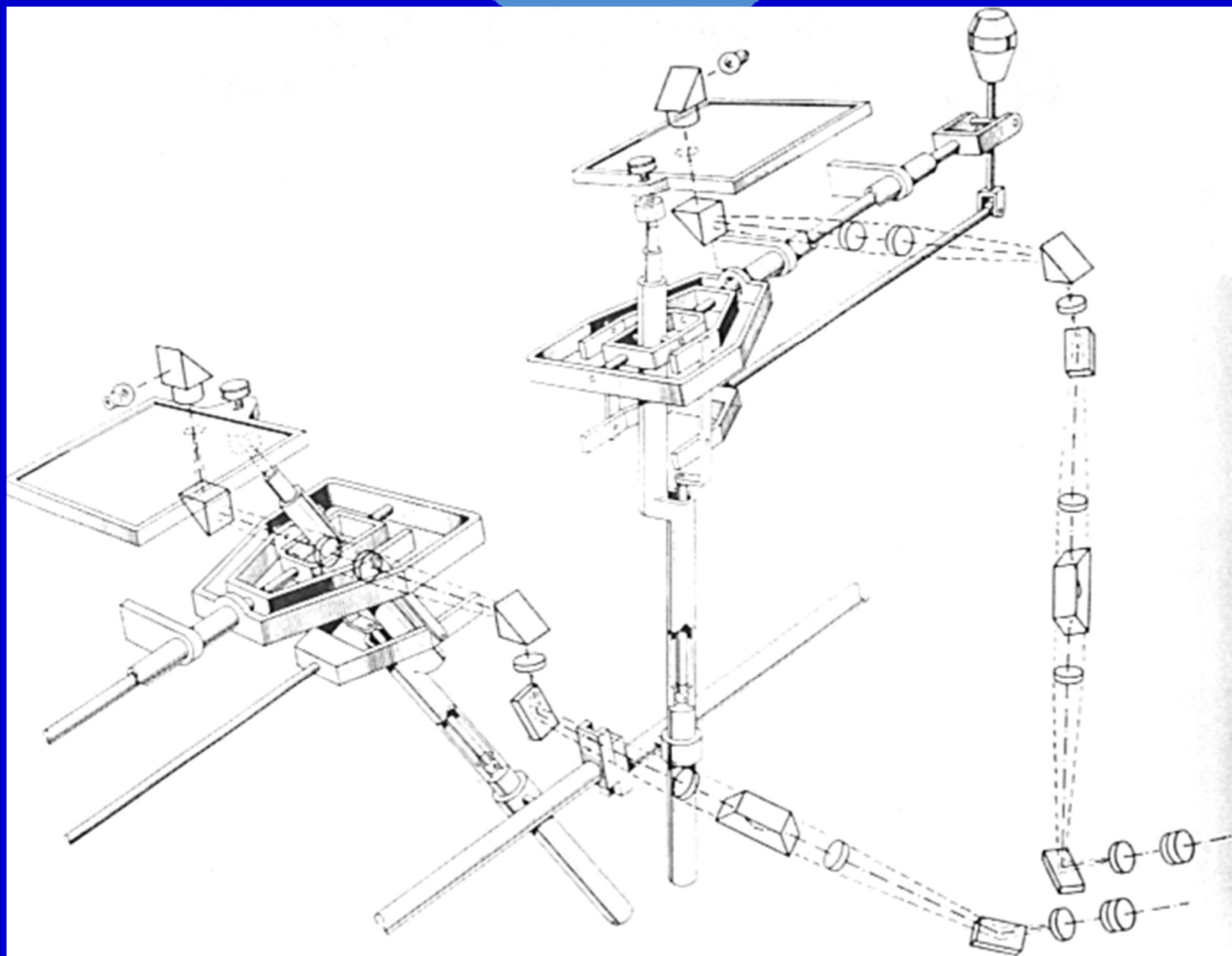
Schema costruttivo dello STEREOSIMPLEX III della GALILEO.
