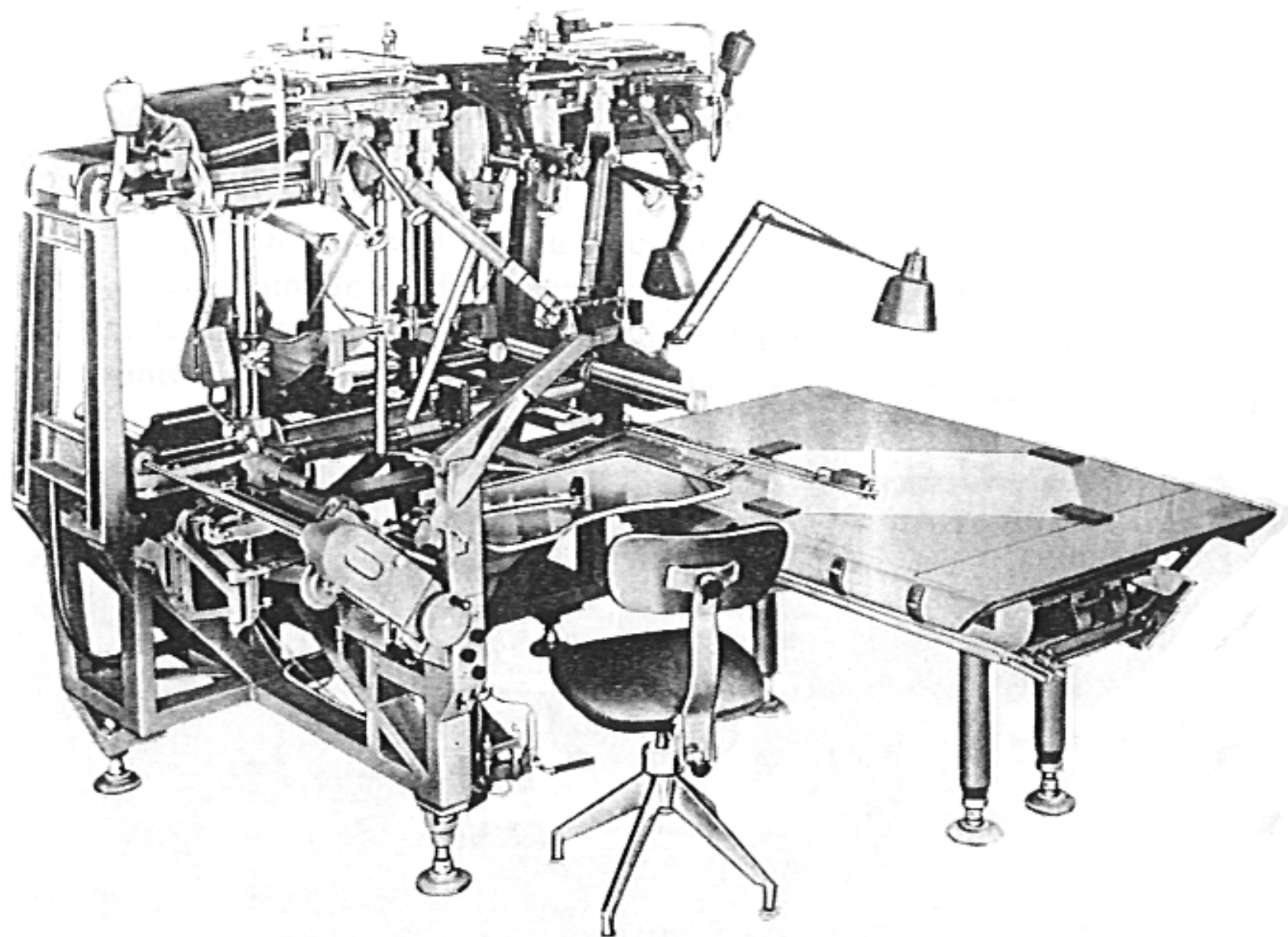
Restitutore STEREOSIMPLEX III della GALILEO.
