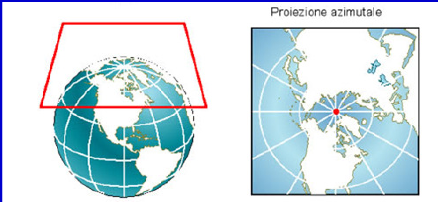
Proiezione azimutale
