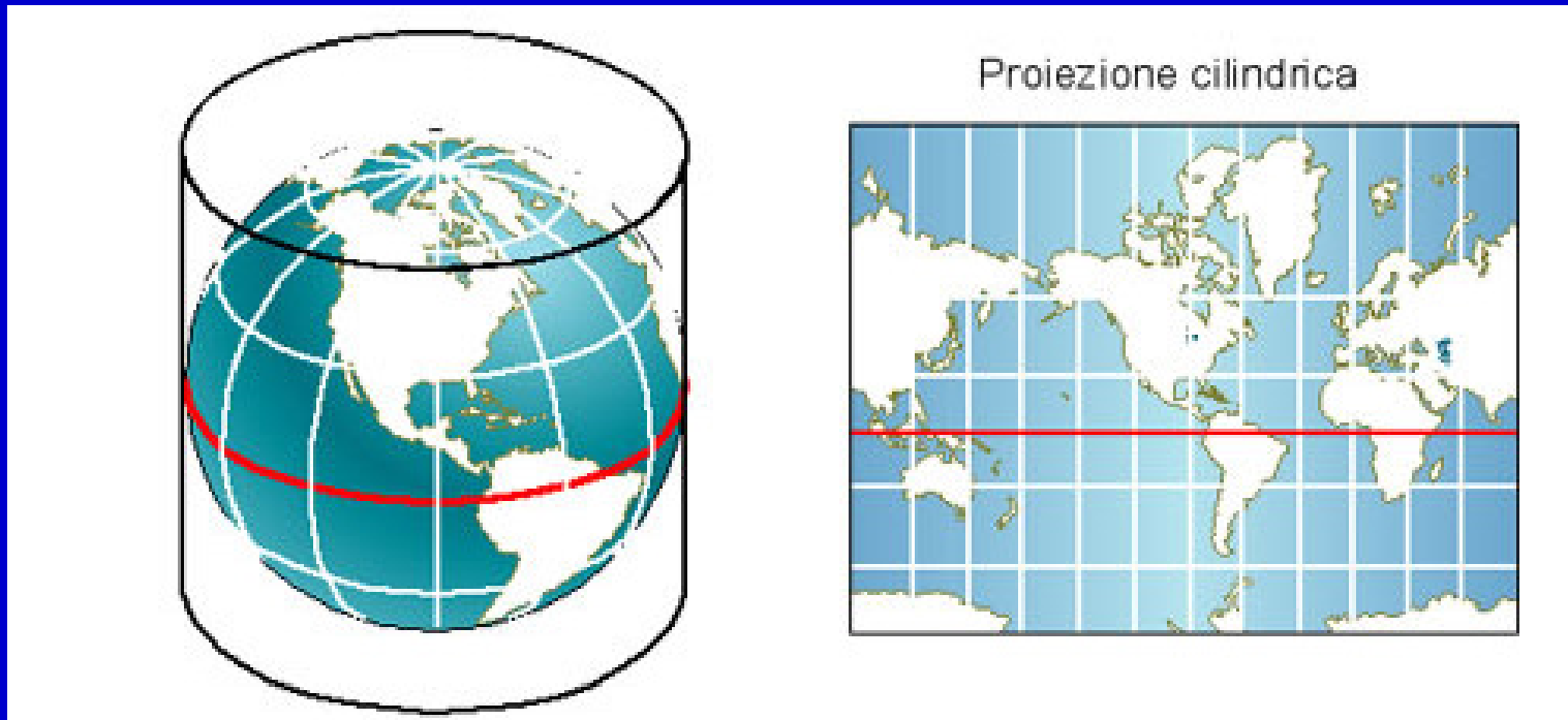
Proiezione cilindrica
