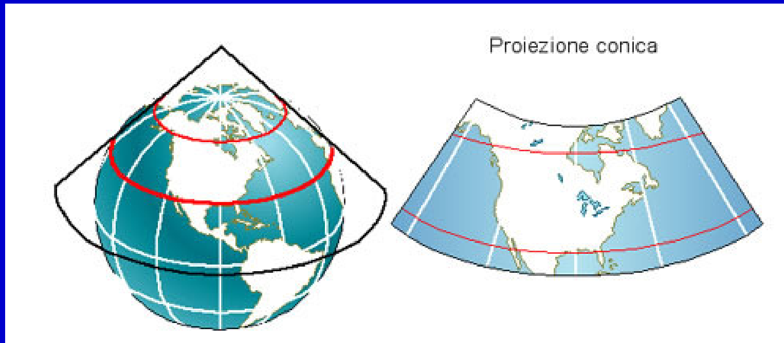
Proiezione conica
